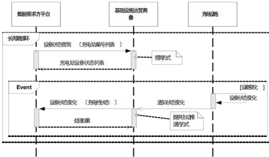
图 A.2 推送设备状态流程
